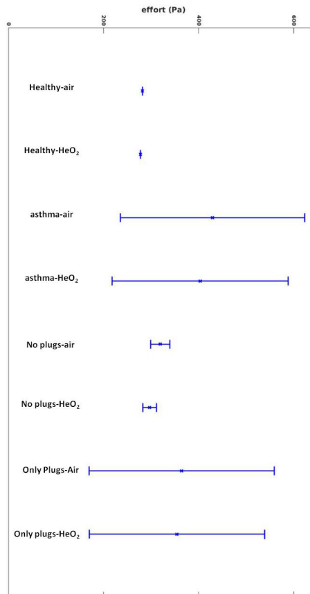
FIGURE 15. Moyennes et écarts-types sur un cycle respiratoire dans différentes configurations : un patient en bonne santé, cinquante configurations d'asthmatiques avec broncho-contractions, cinquante patients avec seulement des broncho-contractions modérées diffuses (plug free) et cinquante patients avec seulement des broncho-contractions importantes isolées (plug uniquement). Comparaison des efforts pour de l'air ou un mélange hélium-oxygène.
