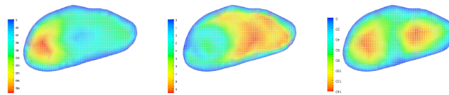
FIGURE 13. Isovaleurs de la vitesse dans le plan de coupe gauche, au maximum de l'inspiration ( t = 0.4s , à gauche), à la transition ( t = 1.6s , au milieu), au maximum de l'expiration ( t = 1.9s , à droite)
