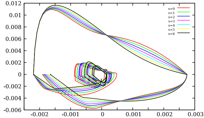
FIGURE 14. Courbes déplacement-débit (en m et \text{m}^3 \cdot \text{s}^{-1} ) pour différentes valeurs de k : k = 40.172 + 10^{s-3} , s = 0, \dots, 6 . La zone des débits positifs correspond à la phase d'expiration et en inspiration les débits sont comptés négativement. Le début de l'expiration se fait au point de volume minimal. Dans une première phase le patient respire normalement, puis inspire profondément, expire et inspire une nouvelle fois.
