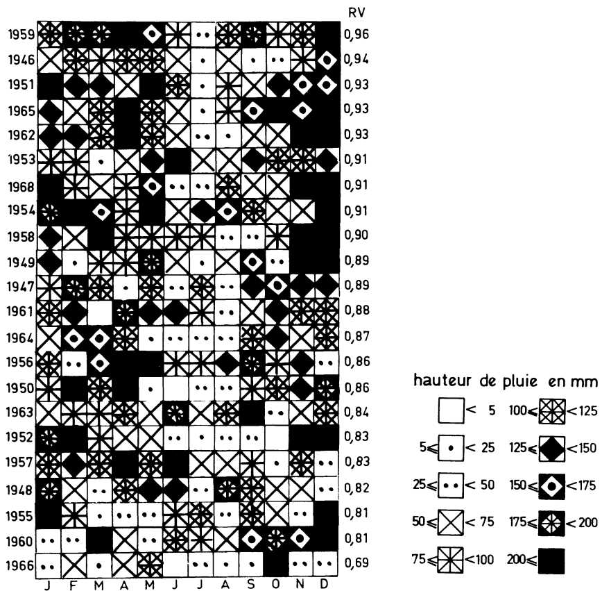
Figure 17 – Arfons-Alzeau, infrastructure, classement des années selon leur coefficient RV.
