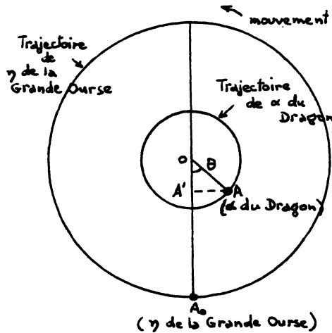
Fig. 2. Position de α du Dragon et de η de la Grande Ourse, à minuit, le 25 juillet de l'an - 2700
