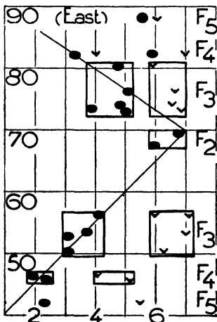
Graphique 3 : Diminution de la grandeur du coefficient de variation (figuré par le signe v) et de la déviation standard (figurée par le signe .), (échelle des valeurs numériques portée en abscisses), en fonction du nombre des autofécondations successives fournissant les générations F_3 , F_4 , F_5 à partir de la F_2 .
