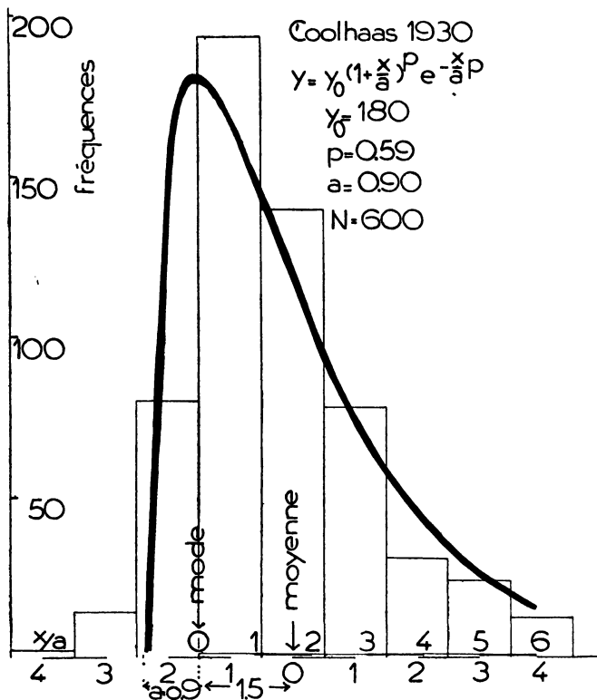
Graphique 4 : Histogramme de distribution des fréquences de la durée de combustion (en secondes) de 600 échantillons de Tabacs (Coolhaas, 1930), son ajustement par la courbe du type III de Pearson (par VEZIAN).
